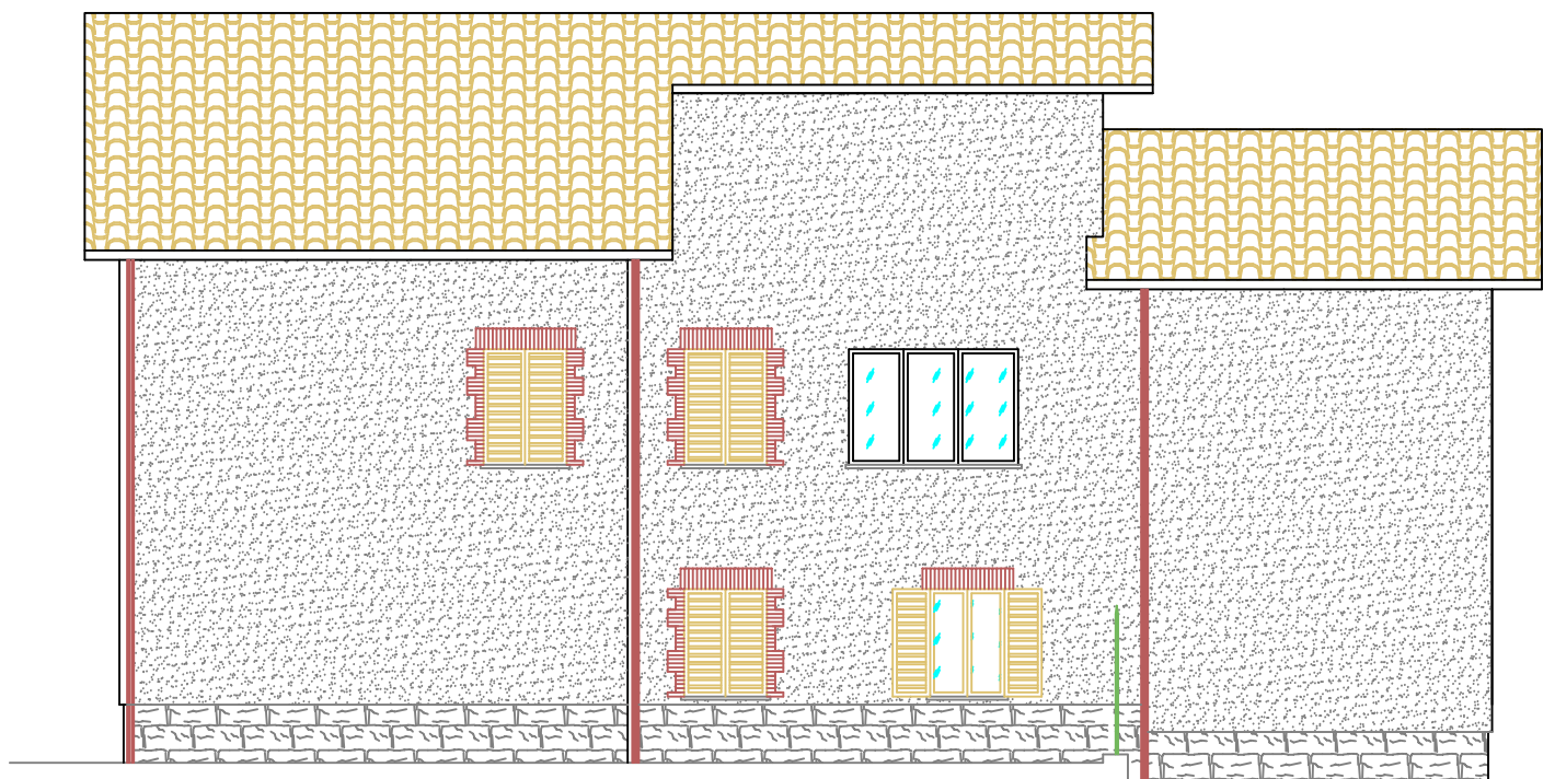
PROSPETTO DX
